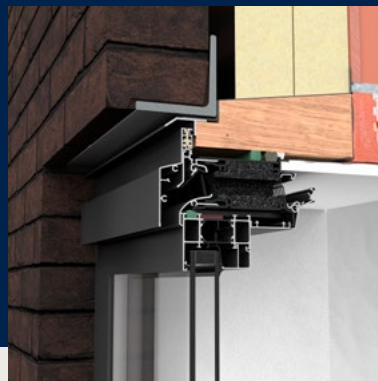
Invisivent®
